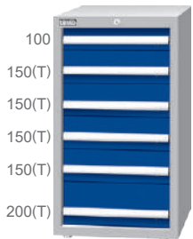
EA-10062(T) W566xD607xH1000 EB-10062(T) W718xD607xH1000 ED-10062(T) W718xD759xH1000
