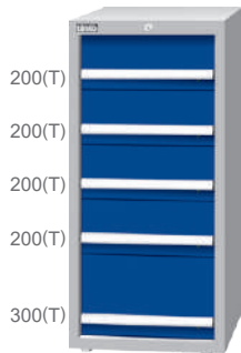
EA-12052(T) W566xD607xH1200 EB-12052(T) W718xD607xH1200 ED-12052(T) W718xD759xH1200
